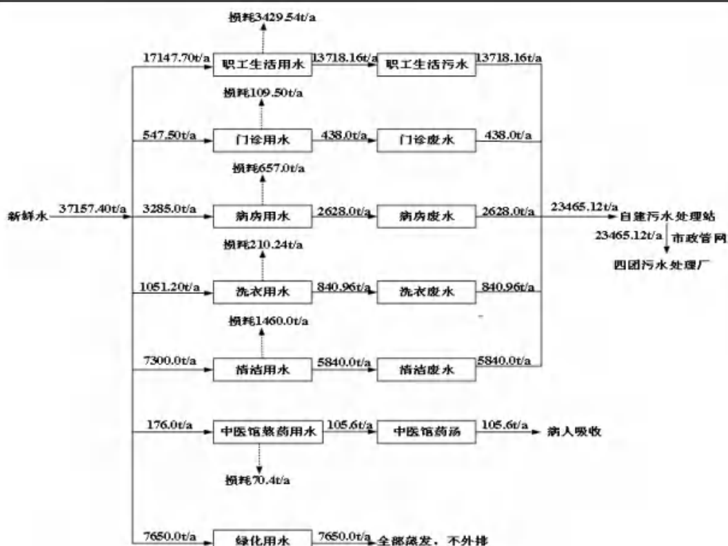
图 2-2-1 本项目水平衡图 (t/a)
