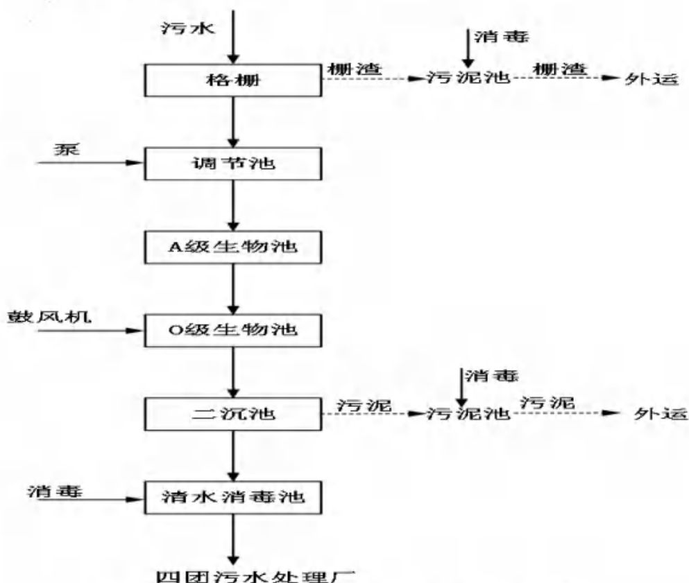
图 2-3 项目自建污水处理站处理工艺及产污环节图
