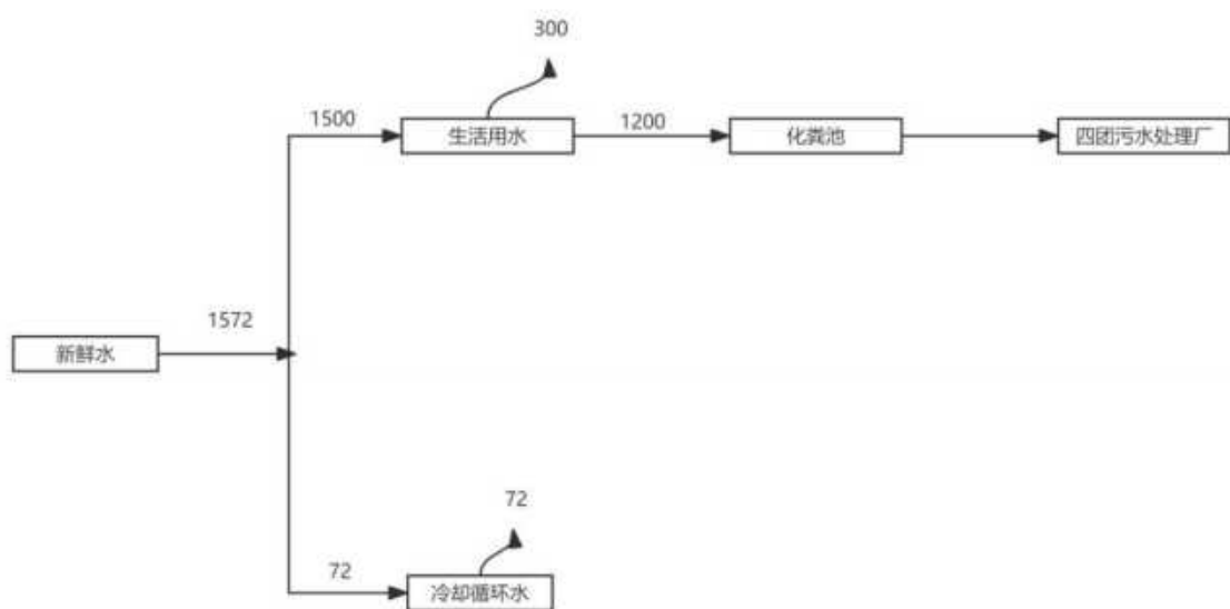
图 2-1 全厂水平衡图 单位: \text{m}^3/\text{a}
