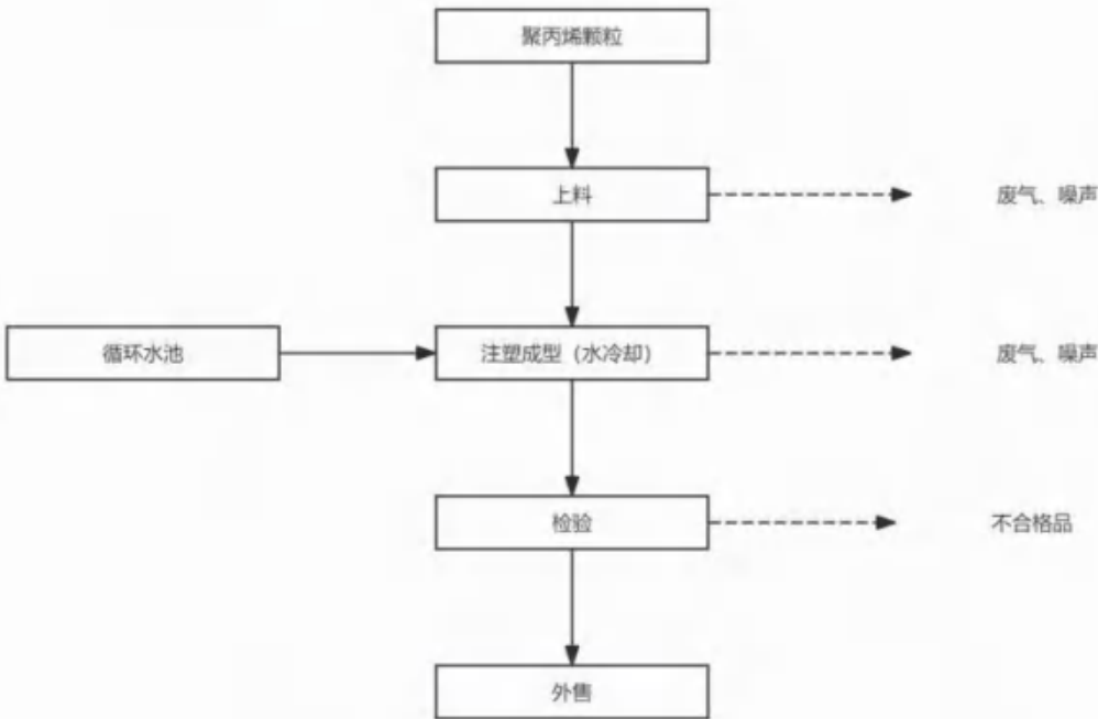
图 2-3 项目运营期生产工艺流程及产污环节示意图
