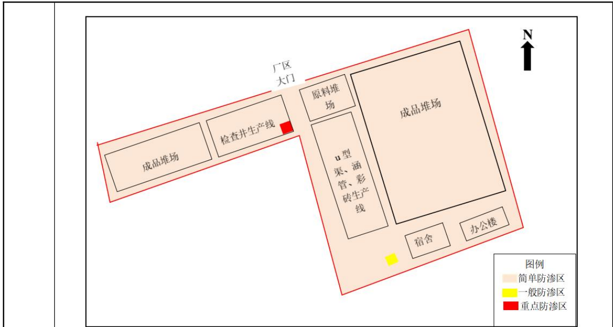
图 4-1 厂区分区防渗图
