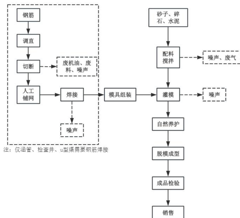
图 2-3 工艺流程图
